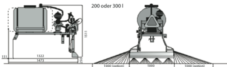
Strahldüsen 0-40km/h
